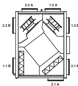
VEX100 - Vertikal LEFT
