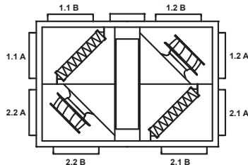
VEX200 - Kompaktfilter Ventilatorplacering 1 - RIGHT
